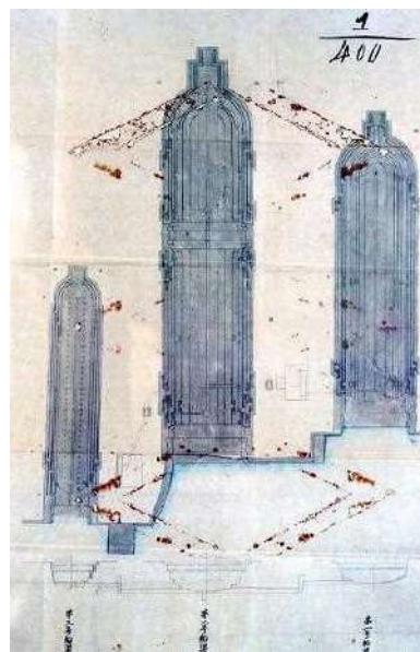
1-12 近代造船所建築図面資料「第一号～第三号船渠配置図」(市博物館蔵)
